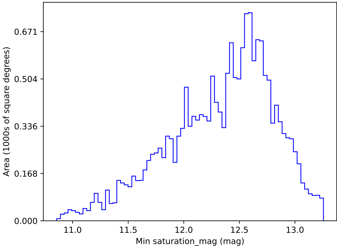
weather_cloudso16v3.4_10yrs WFD r band: Min saturation_mag
