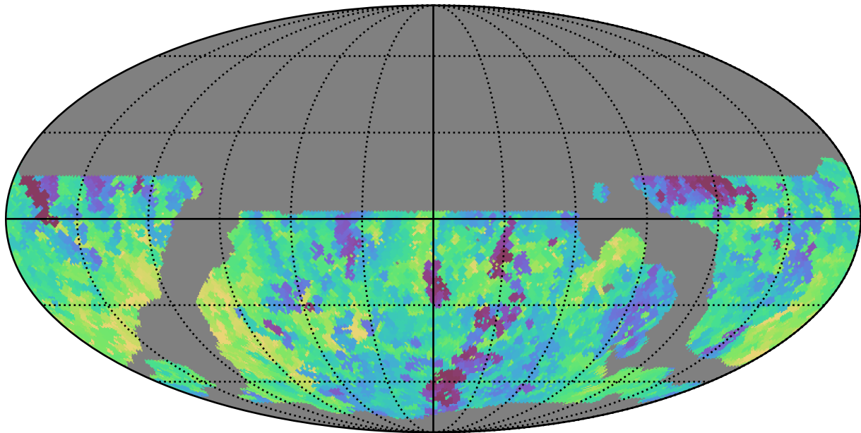
weather_cloudso16v3.4_10yrs WFD i band: Min saturation_mag
