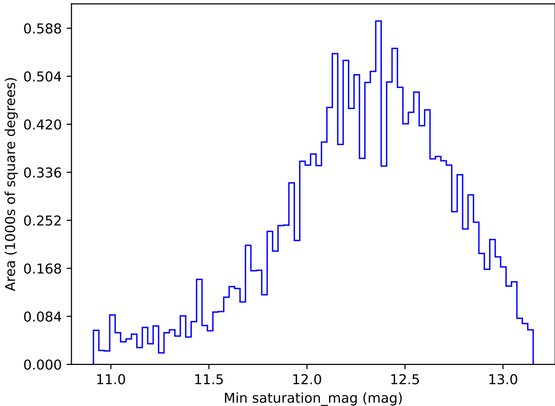
weather_cloudso16v3.4_10yrs WFD i band: Min saturation_mag
