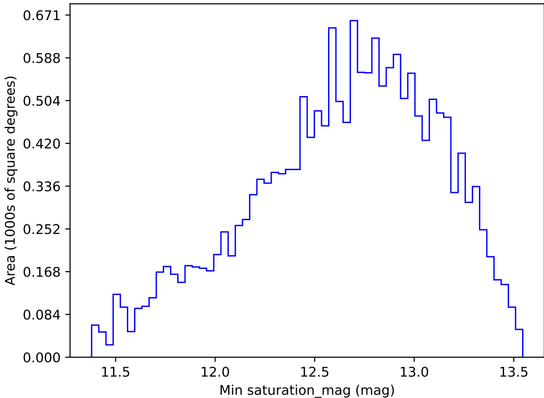
weather_cloudso16v3.4_10yrs WFD g band: Min saturation_mag
