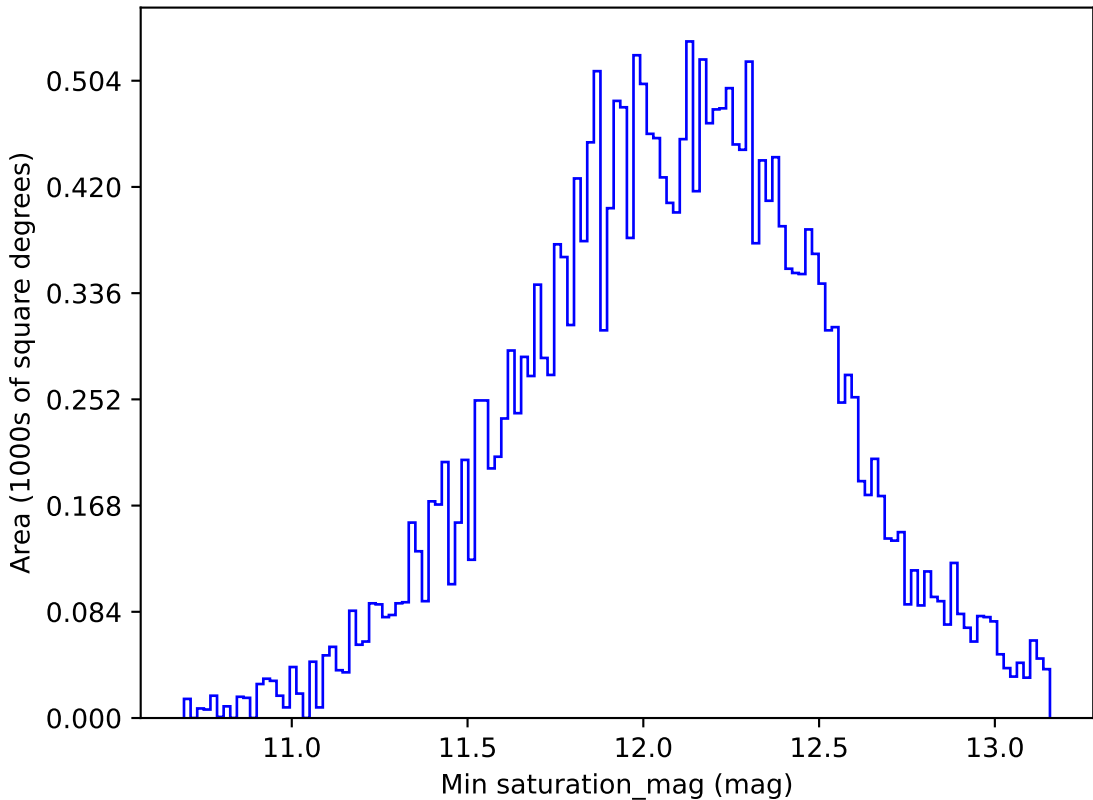
weather_cloudso16v3.4_10yrs All sky z band: Min saturation_mag
