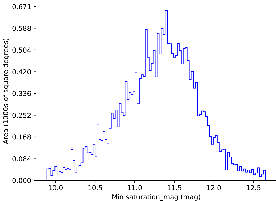
weather_cloudso16v3.4_10yrs All sky u band: Min saturation_mag
