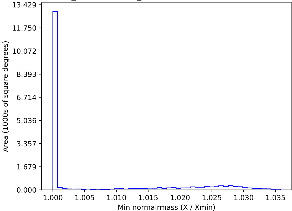
weather_cloudso16v3.4_10yrs WFD z band: Min normairmass
