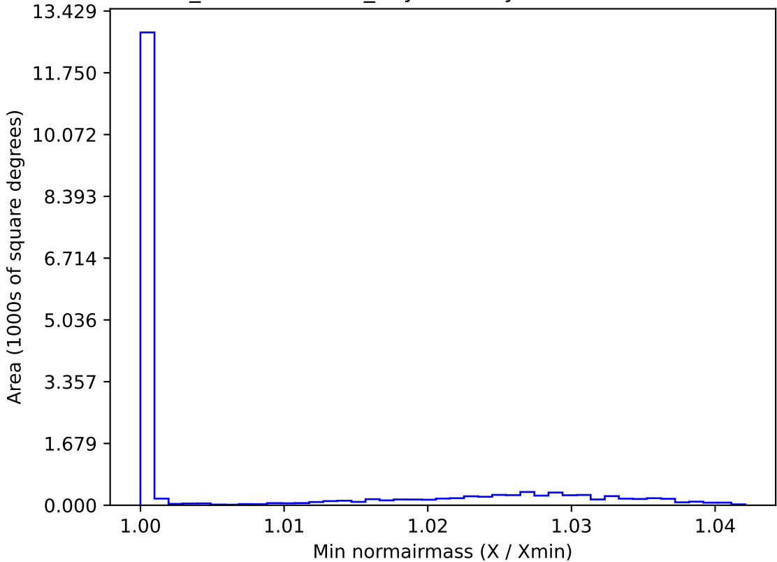
weather_cloudso16v3.4_10yrs WFD y band: Min normairmass
