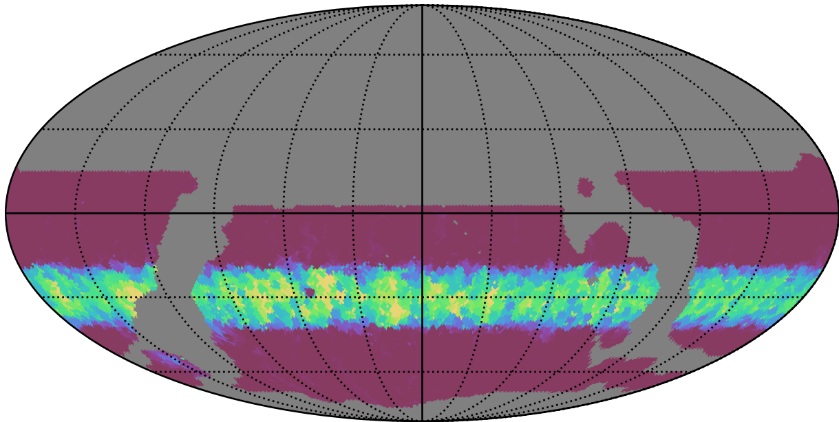
weather_cloudso16v3.4_10yrs WFD u band: Min normairmass
