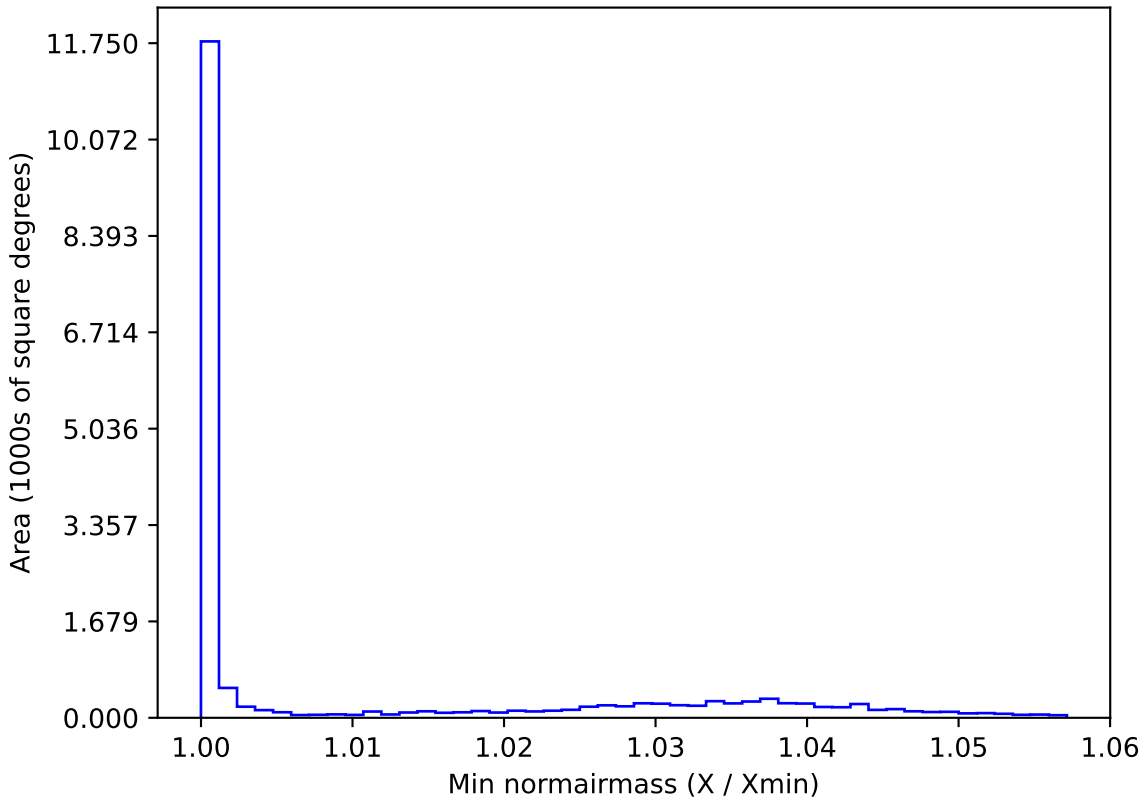
weather_cloudso16v3.4_10yrs WFD u band: Min normairmass
