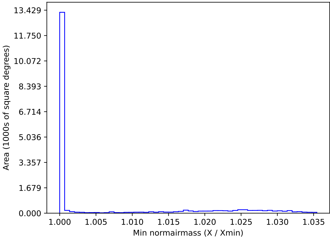
weather_cloudso16v3.4_10yrs WFD r band: Min normairmass
