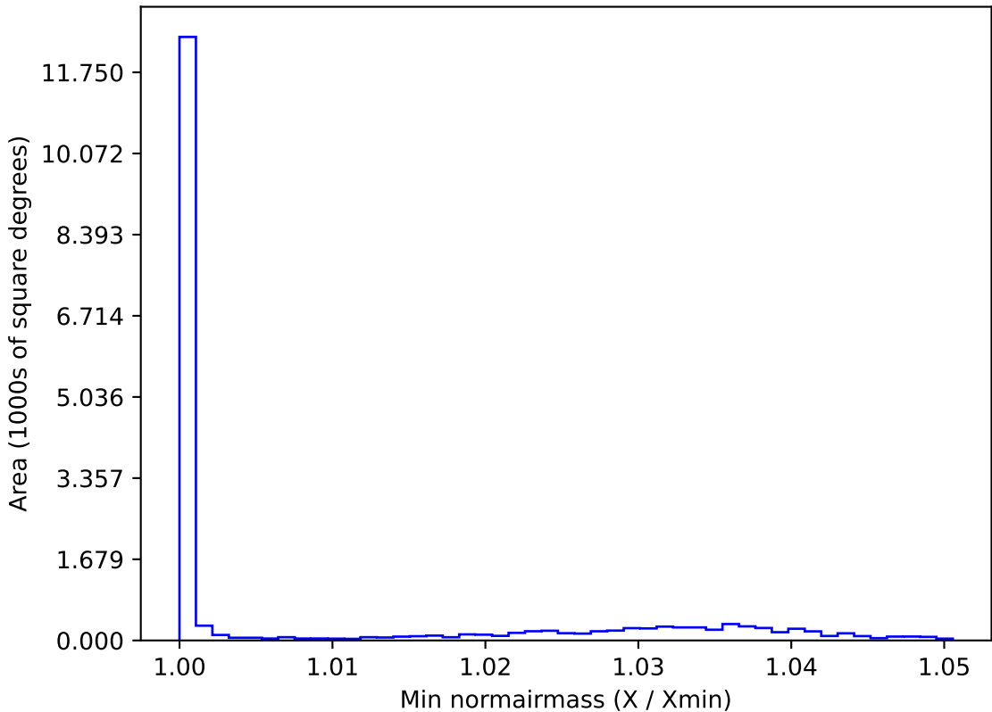
weather_cloudso16v3.4_10yrs WFD g band: Min normairmass
