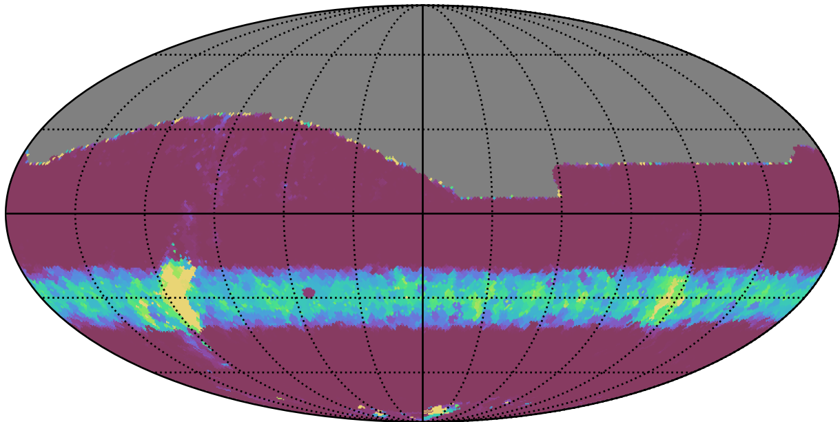
weather_cloudso16v3.4_10yrs All sky z band: Min normairmass
