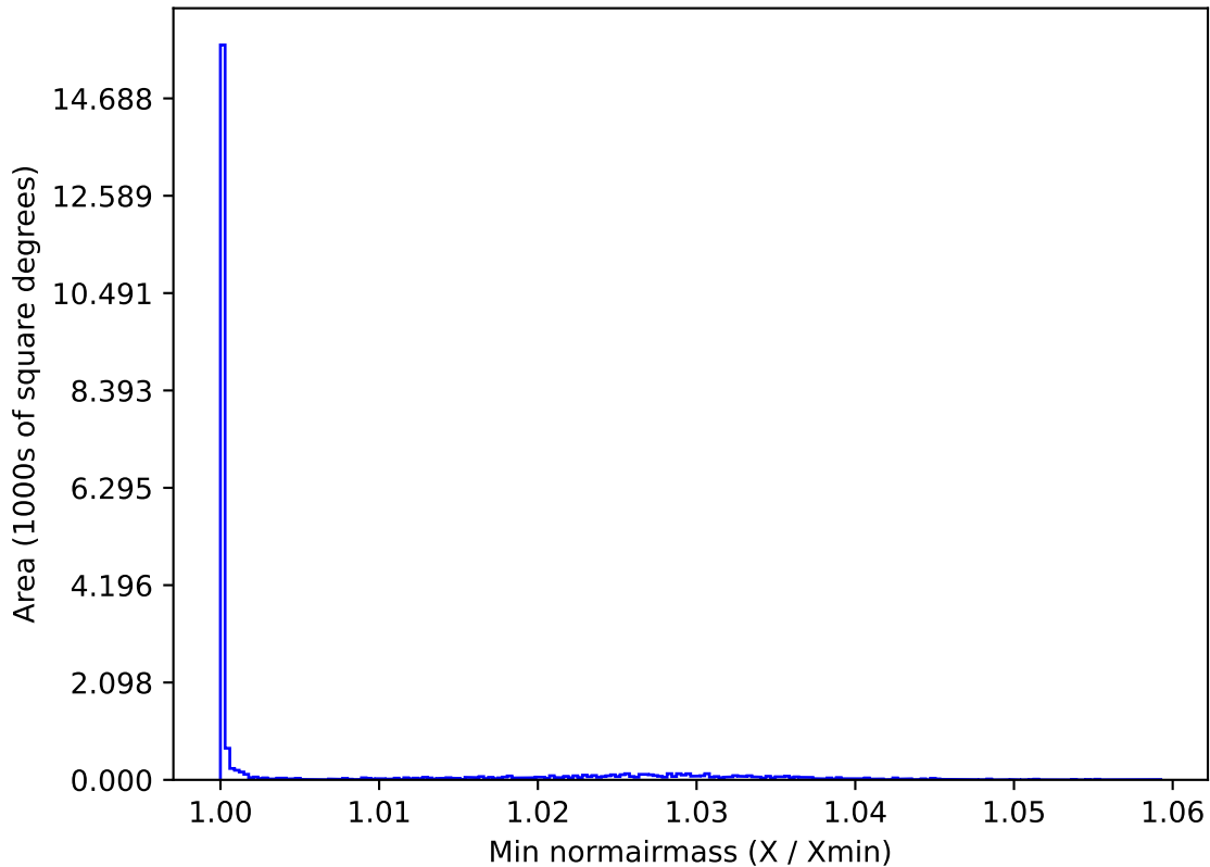
weather_cloudso16v3.4_10yrs All sky y band: Min normairmass
