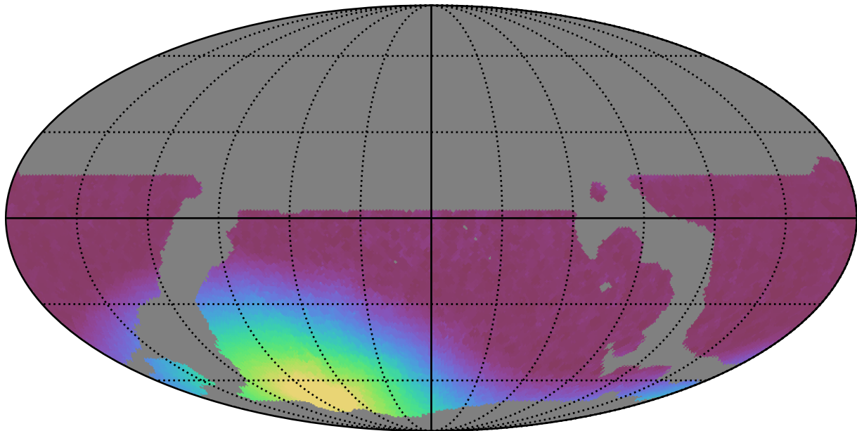
weather_cloudso16v3.4_10yrs WFD y band: Min moonDistance
