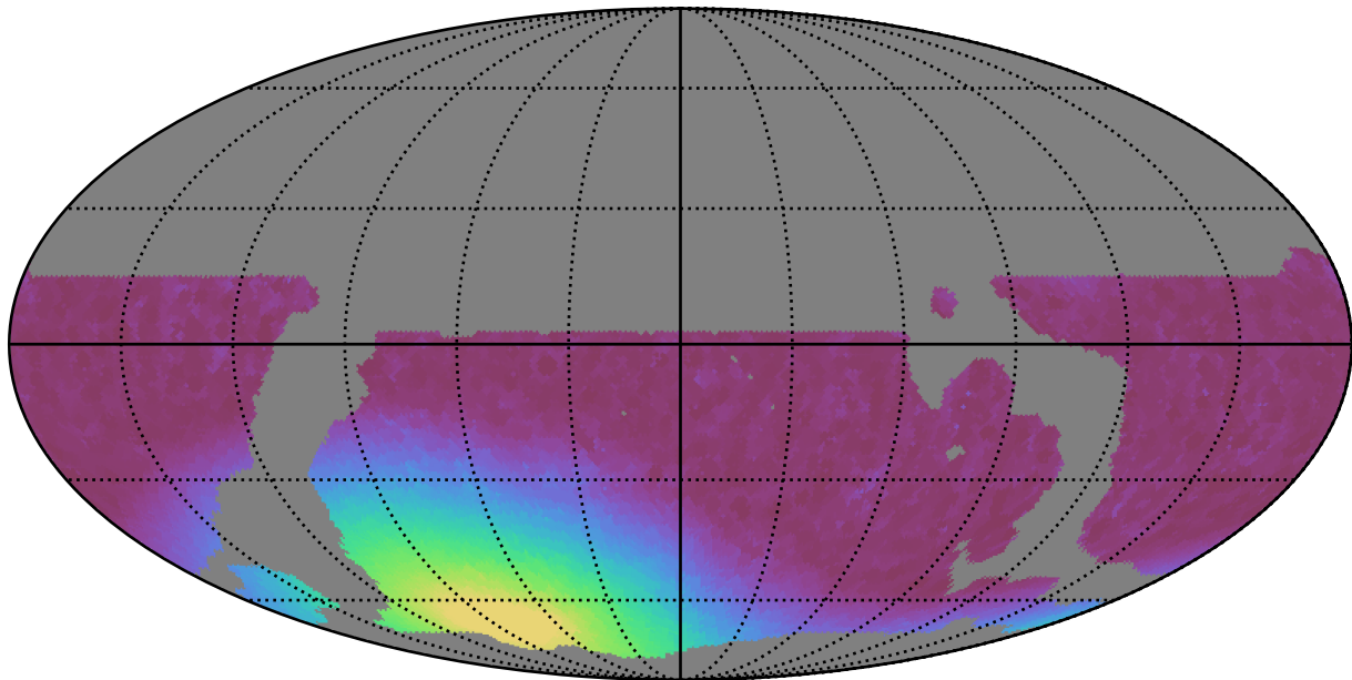
weather_cloudso16v3.4_10yrs WFD i band: Min moonDistance
