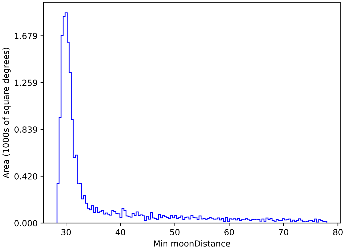
weather_cloudso16v3.4_10yrs WFD i band: Min moonDistance
