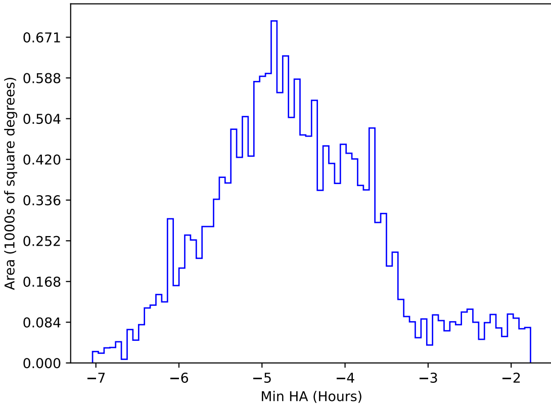
weather_cloudso16v3.4_10yrs WFD z band: Min HA
