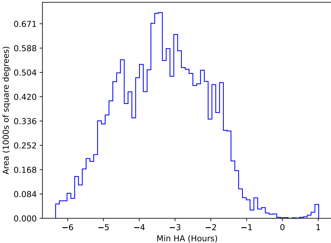
weather_cloudso16v3.4_10yrs WFD u band: Min HA
