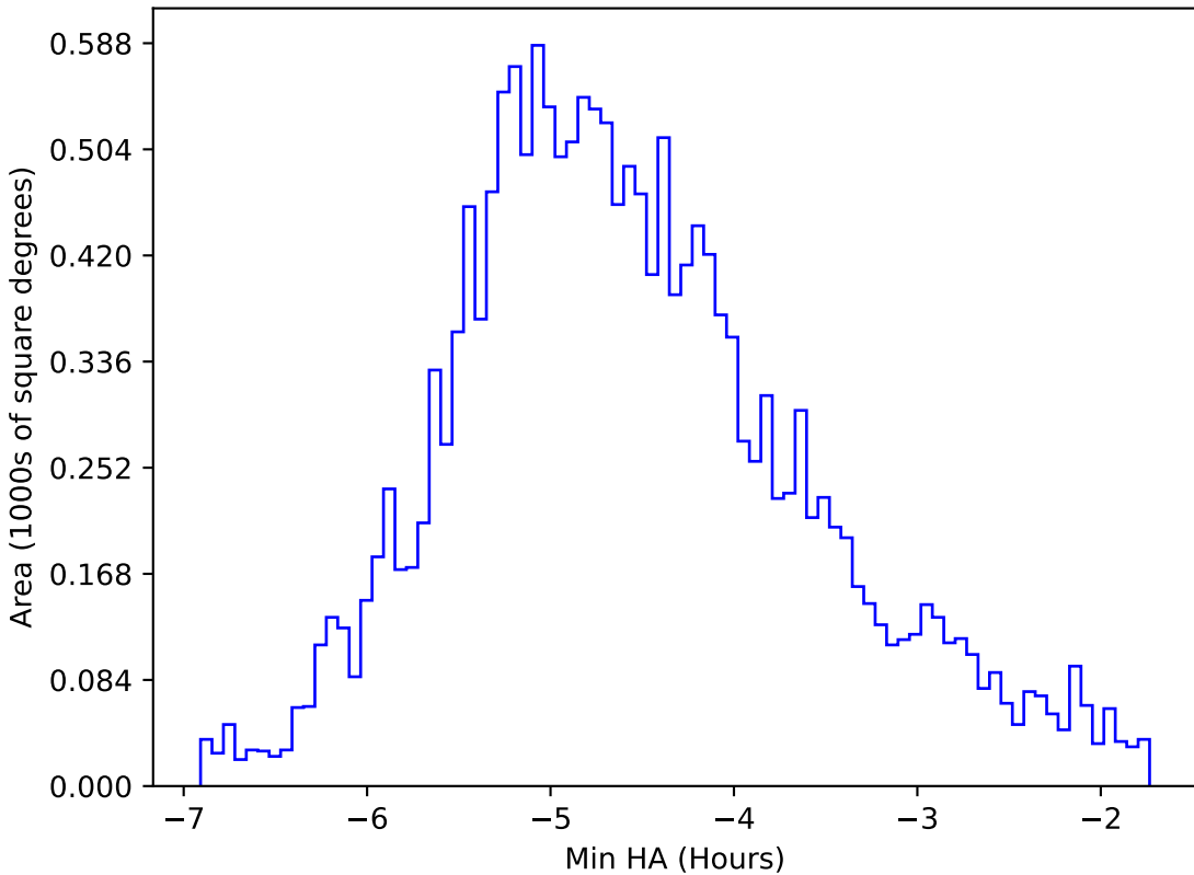
weather_cloudso16v3.4_10yrs WFD r band: Min HA
