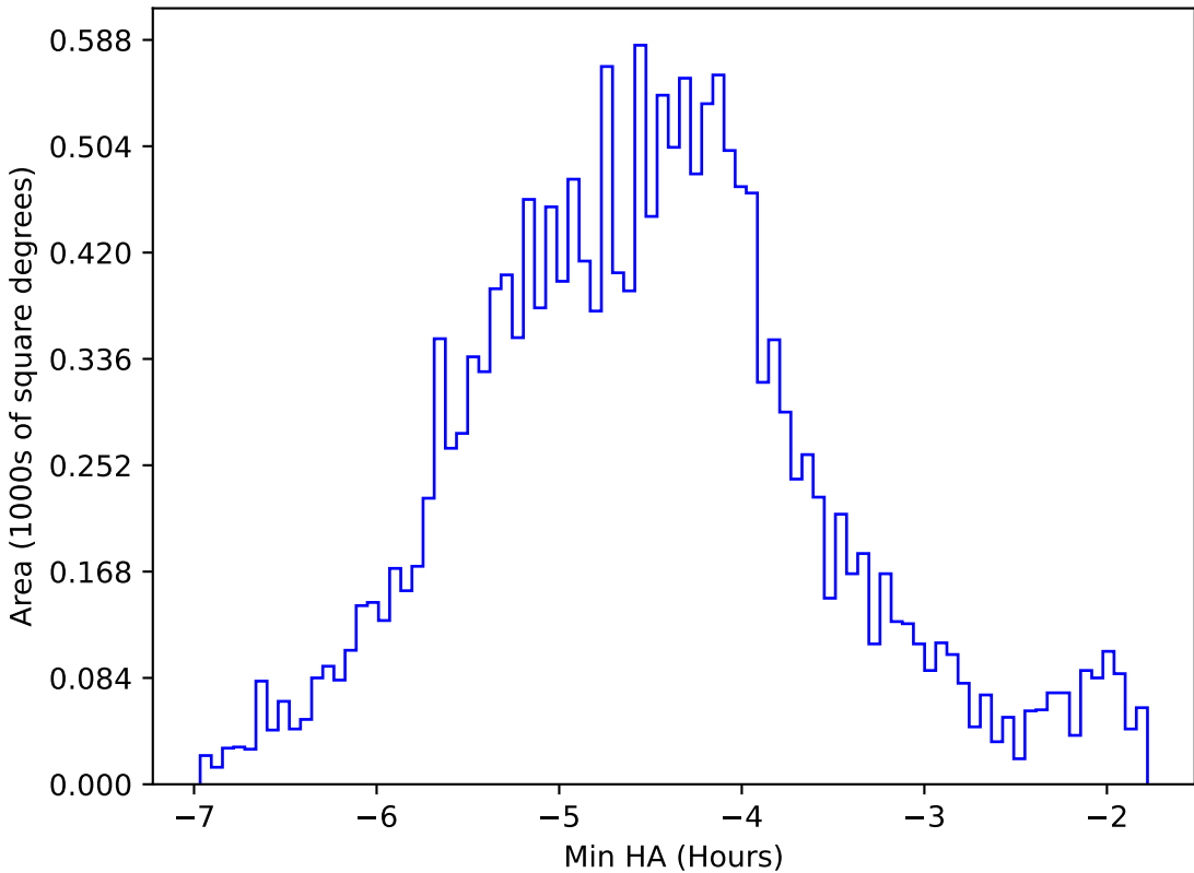
weather_cloudso16v3.4_10yrs WFD i band: Min HA
