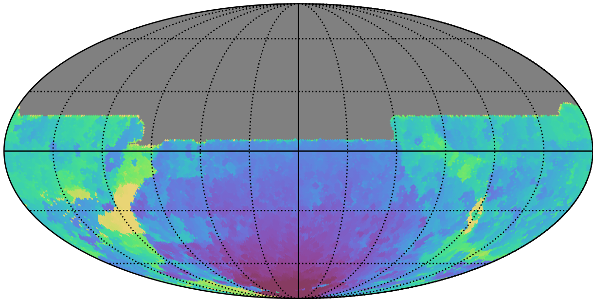
weather_cloudso16v3.4_10yrs All sky y band: Min HA
