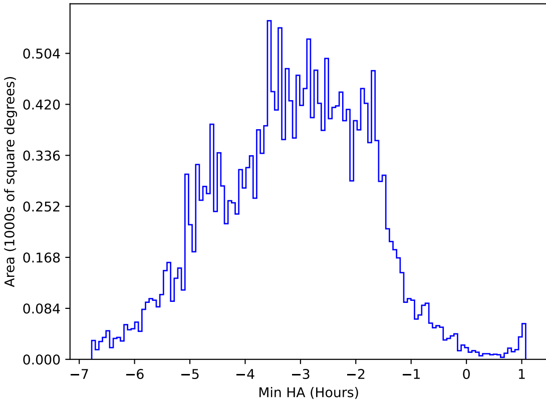
weather_cloudso16v3.4_10yrs All sky u band: Min HA
