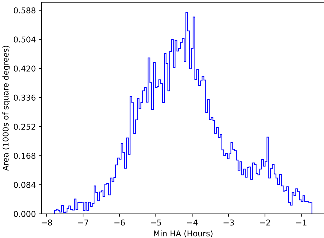
weather_cloudso16v3.4_10yrs All sky i band: Min HA
