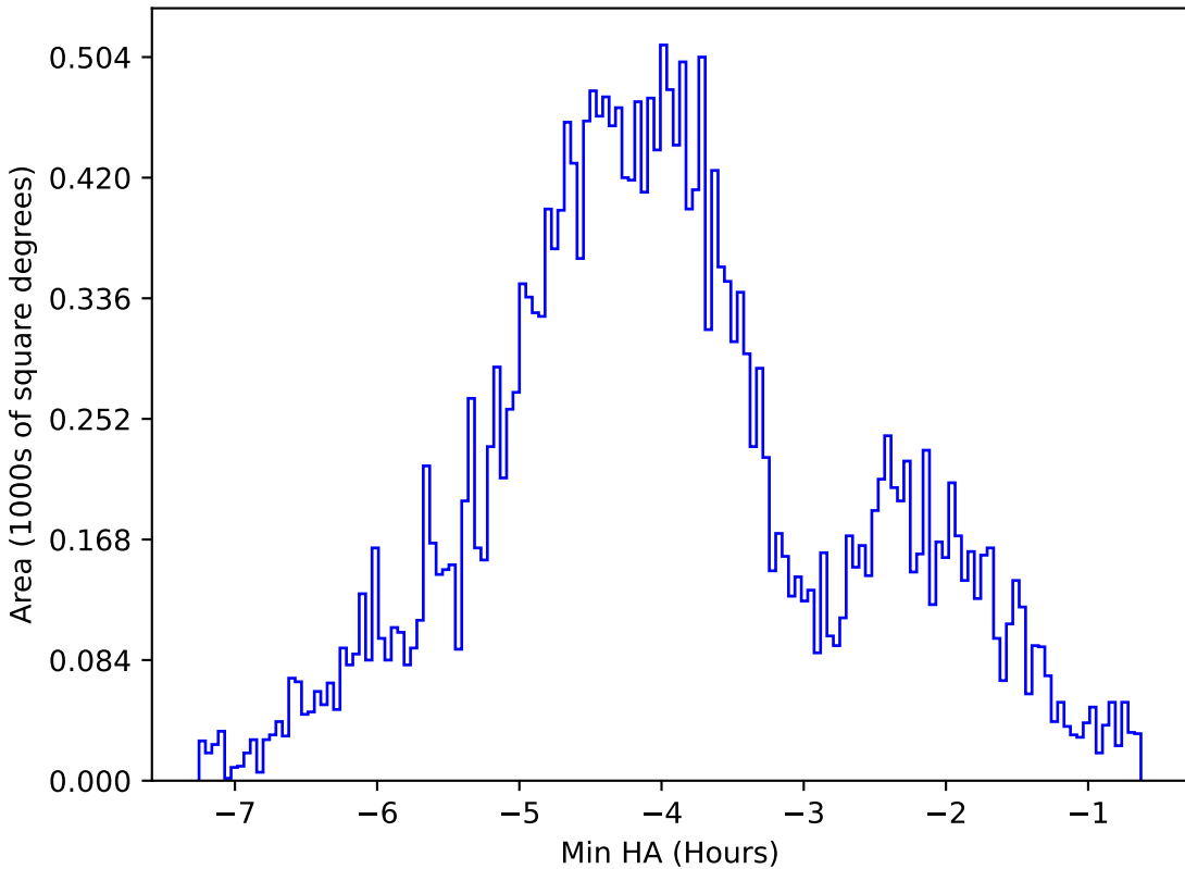
weather_cloudso16v3.4_10yrs All sky g band: Min HA
