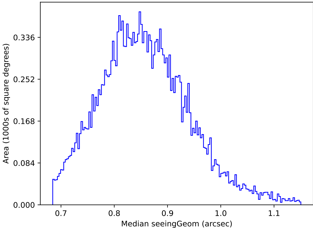
weather_cloudso16v3.4_10yrs Yr 1 y band: Median seeingGeom
