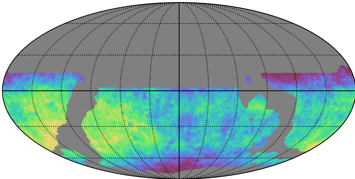
weather_cloudso16v3.4_10yrs WFD z band: Median saturation_mag
