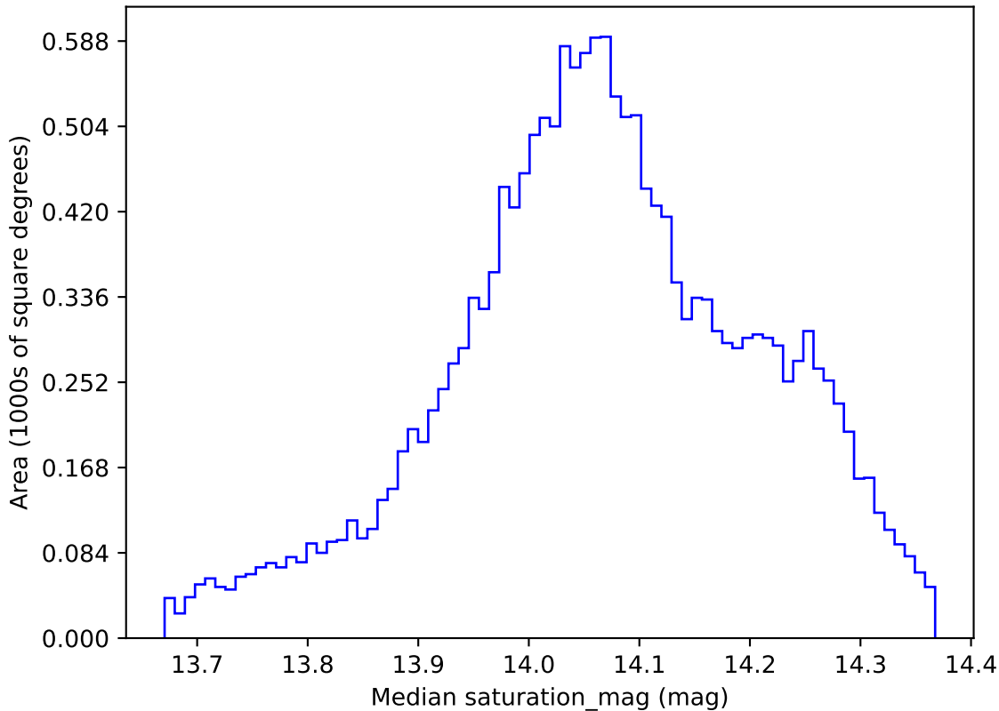
weather_cloudso16v3.4_10yrs WFD z band: Median saturation_mag
