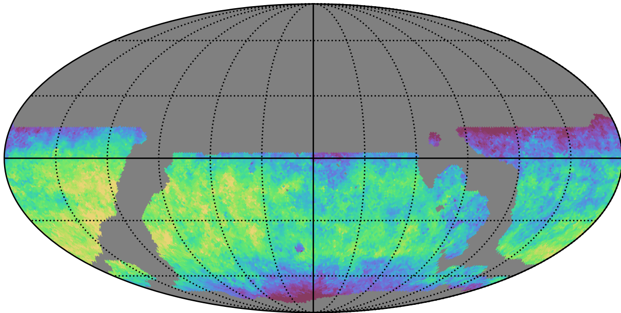
weather_cloudso16v3.4_10yrs WFD y band: Median saturation_mag
