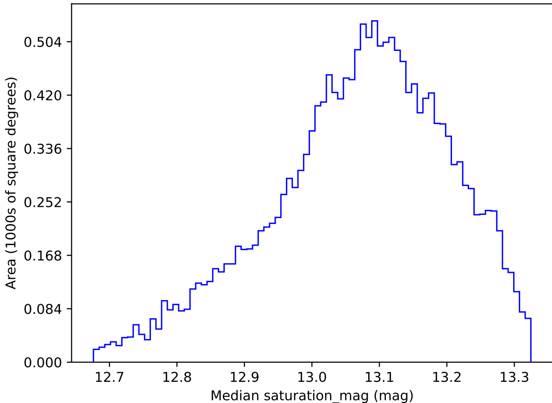
weather_cloudso16v3.4_10yrs WFD y band: Median saturation_mag
