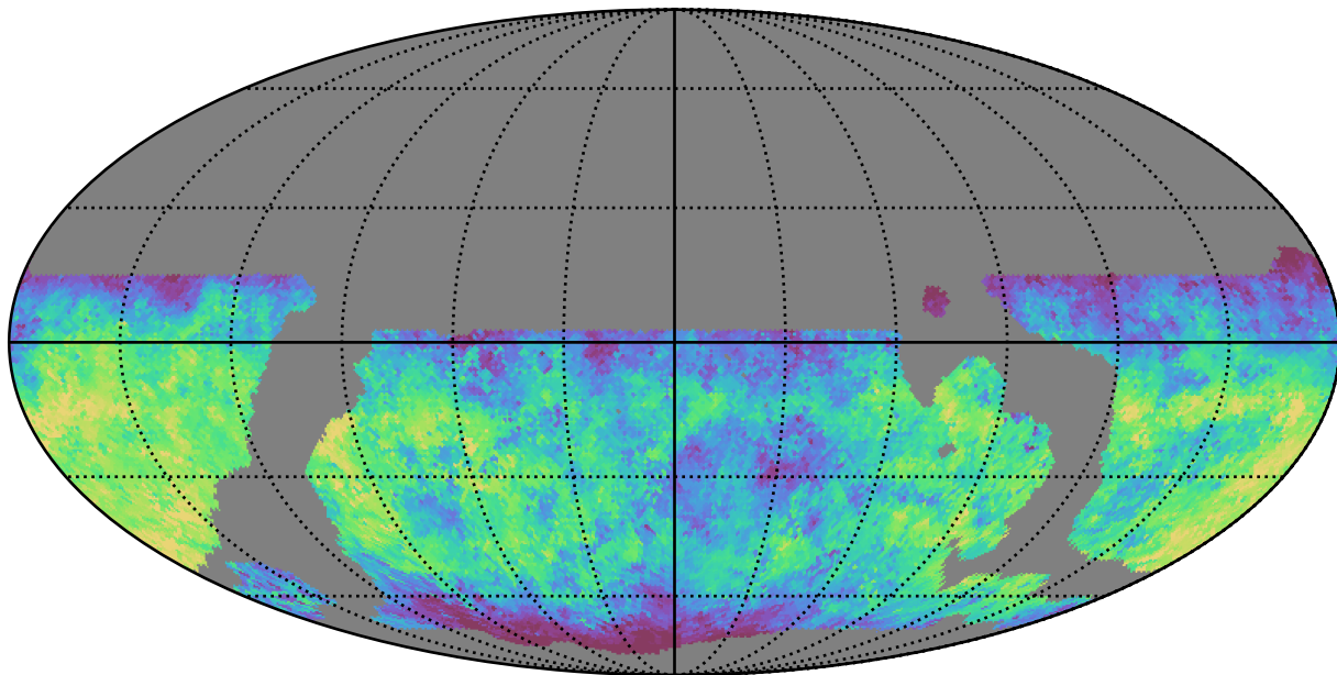
weather_cloudso16v3.4_10yrs WFD u band: Median saturation_mag
