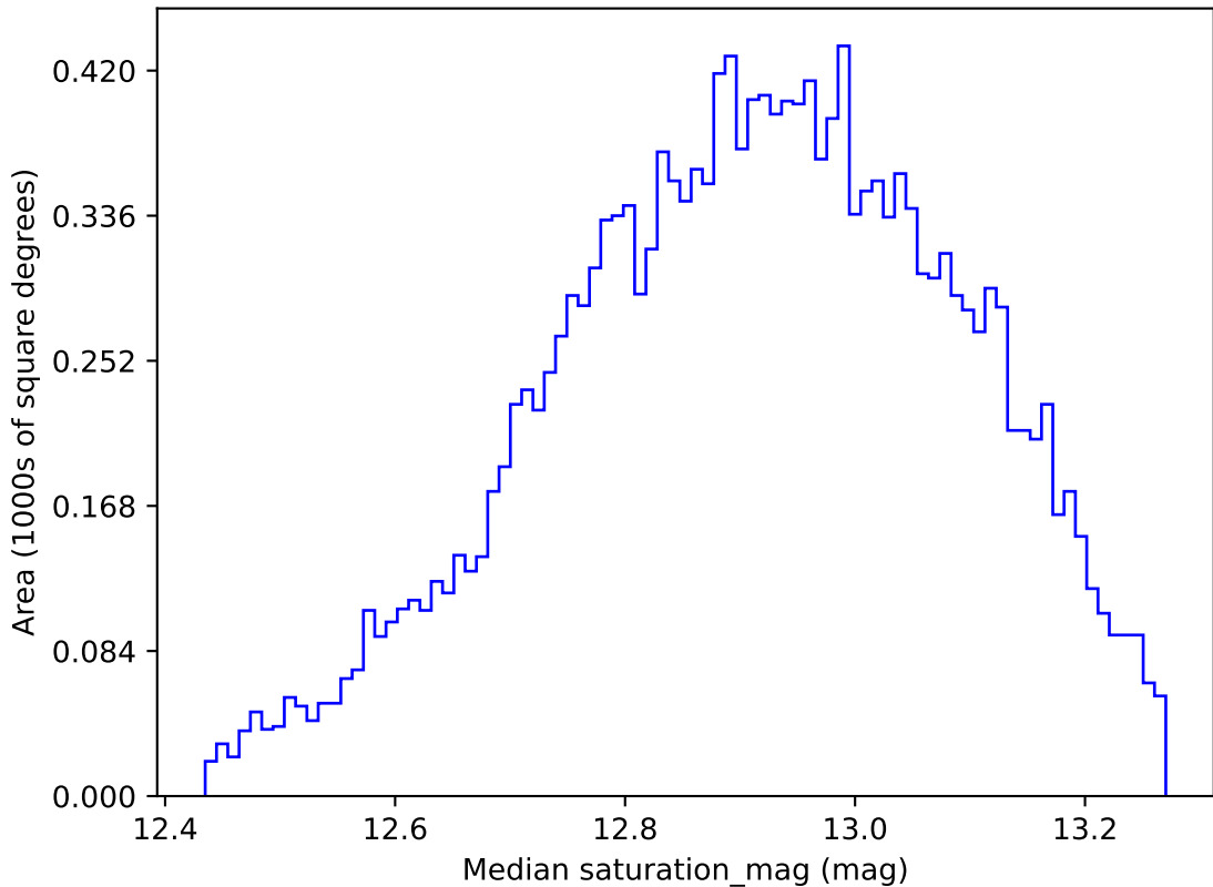
weather_cloudso16v3.4_10yrs WFD u band: Median saturation_mag
