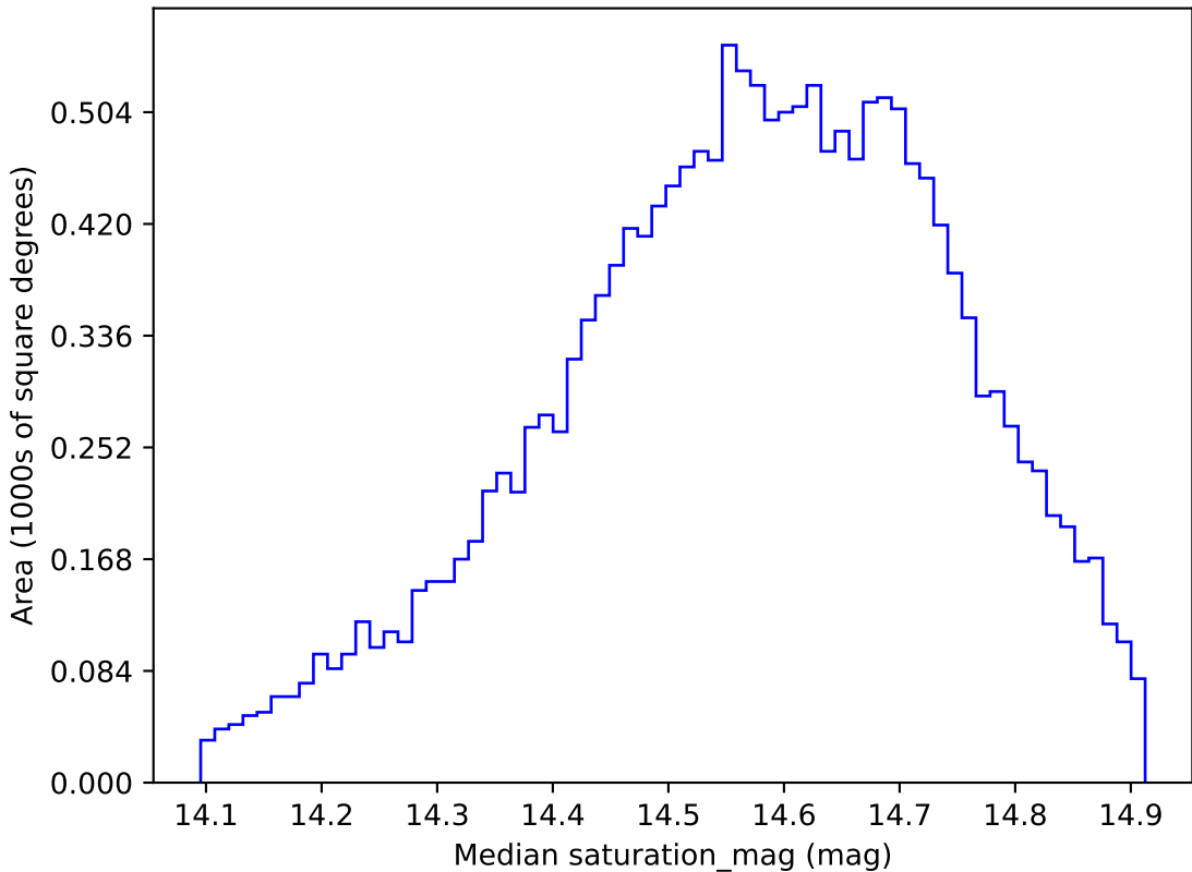
weather_cloudso16v3.4_10yrs WFD r band: Median saturation_mag
