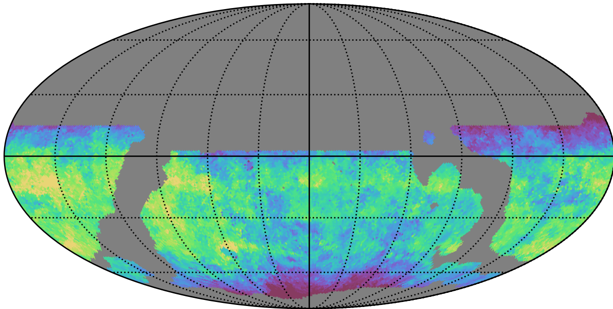
weather_cloudso16v3.4_10yrs WFD g band: Median saturation_mag
