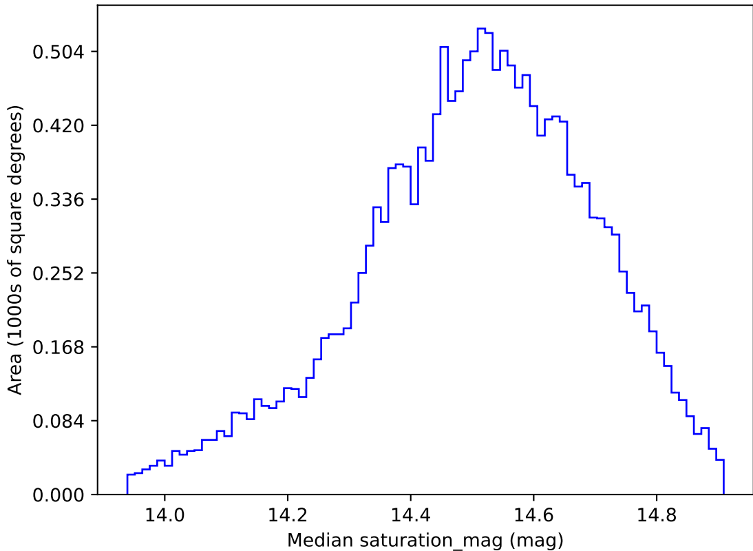
weather_cloudso16v3.4_10yrs WFD g band: Median saturation_mag
