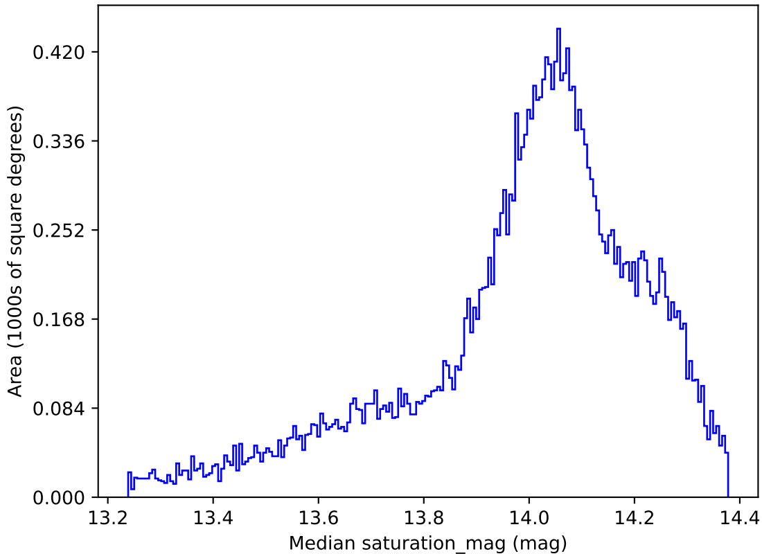
weather_cloudso16v3.4_10yrs All sky z band: Median saturation_mag
