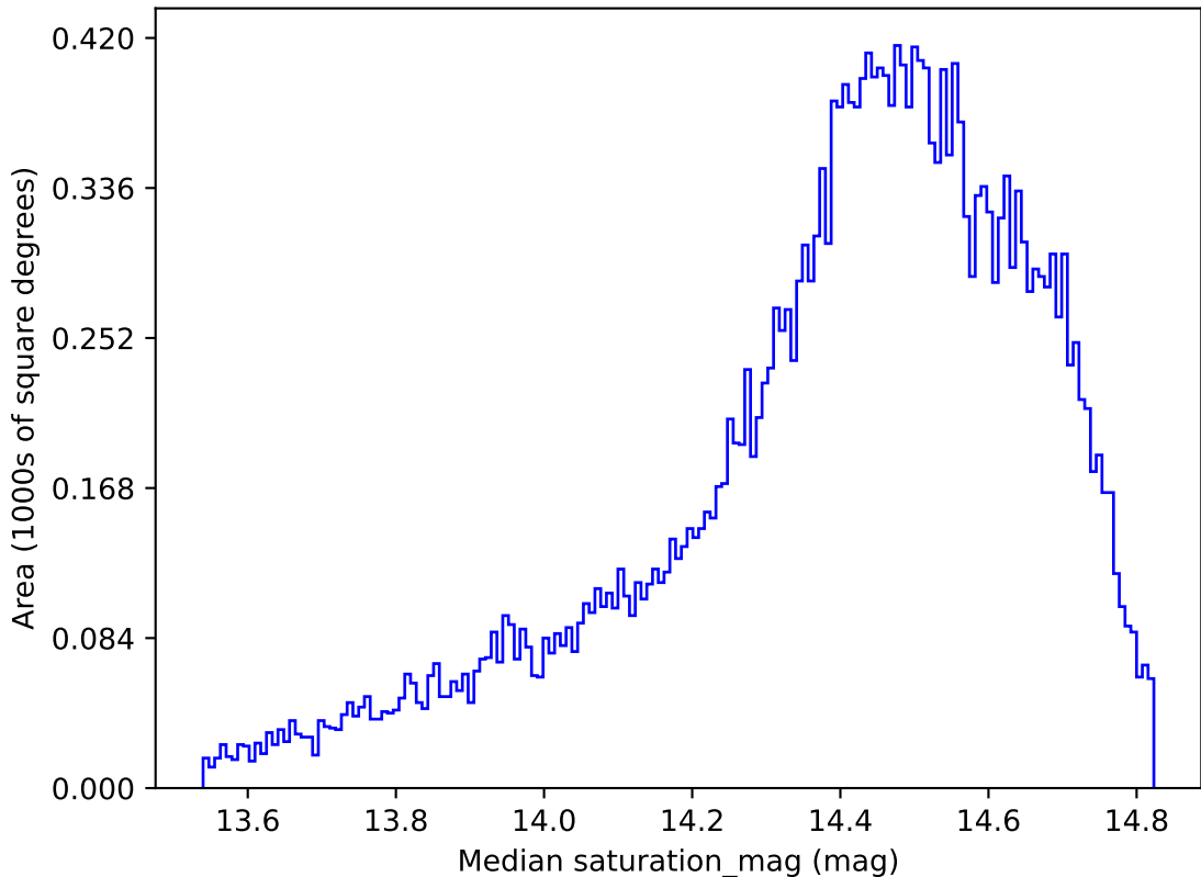
weather_cloudso16v3.4_10yrs All sky i band: Median saturation_mag
