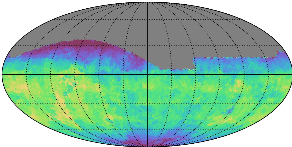
weather_cloudso16v3.4_10yrs All sky g band: Median saturation_mag
