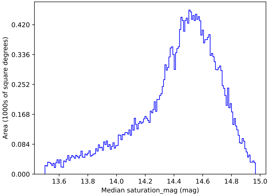
weather_cloudso16v3.4_10yrs All sky g band: Median saturation_mag
