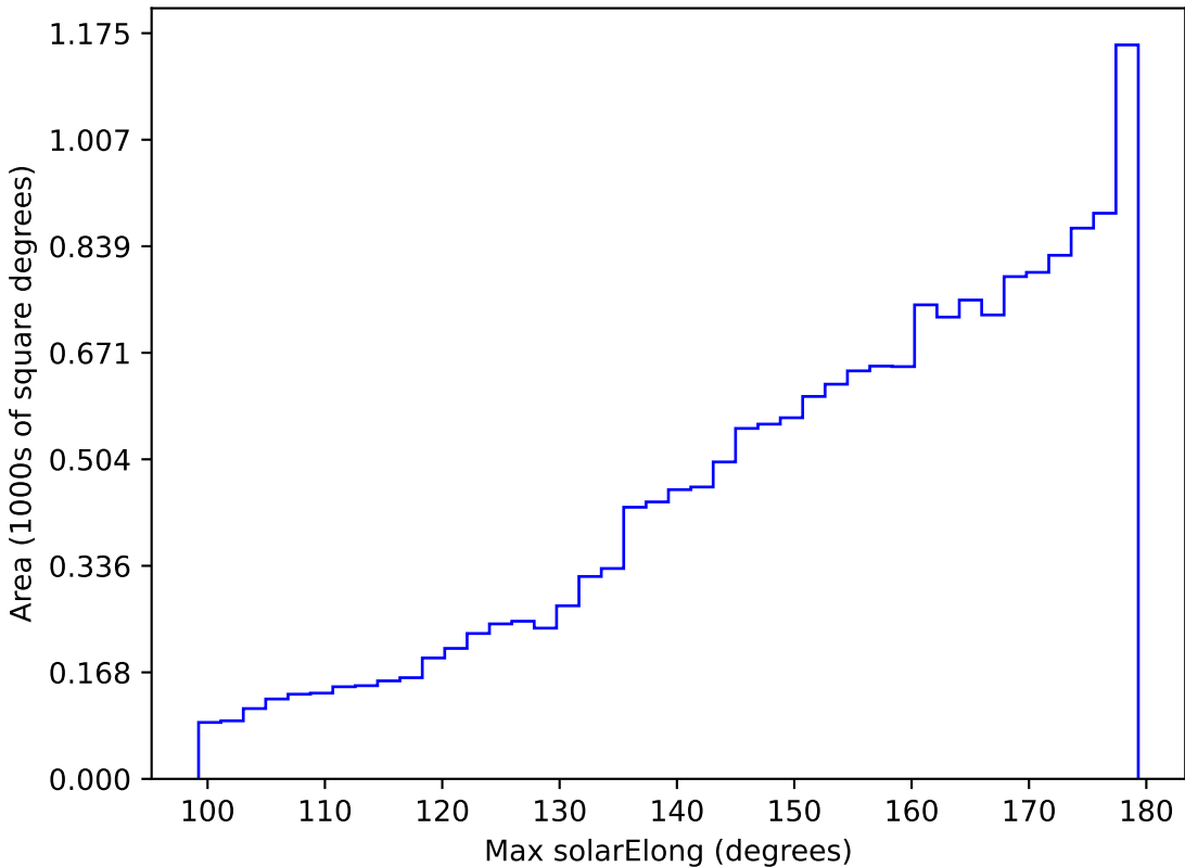
weather_cloudso16v3.4_10yrs WFD z band: Max solarElong
