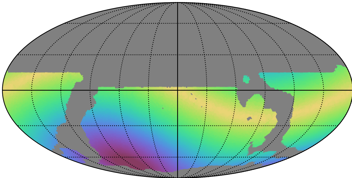
weather_cloudso16v3.4_10yrs WFD y band: Max solarElong
