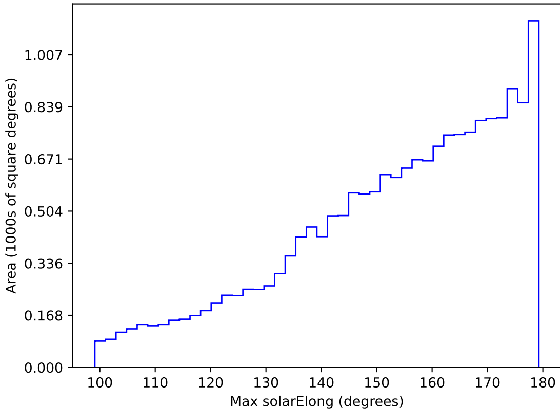
weather_cloudso16v3.4_10yrs WFD y band: Max solarElong
