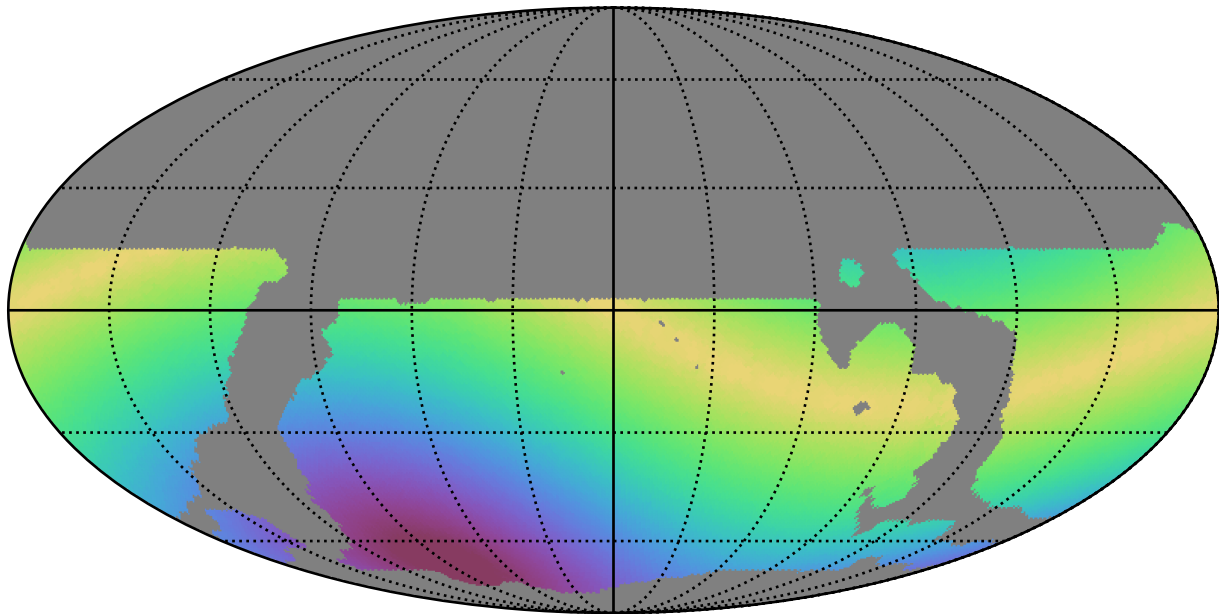
weather_cloudso16v3.4_10yrs WFD i band: Max solarElong
