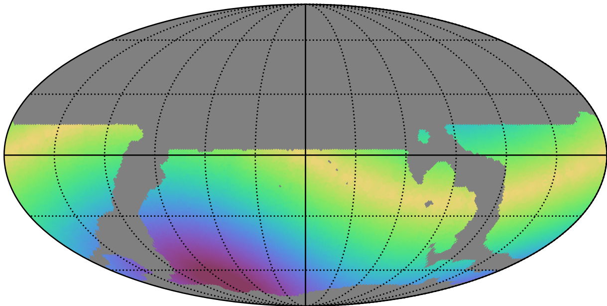
weather_cloudso16v3.4_10yrs WFD g band: Max solarElong
