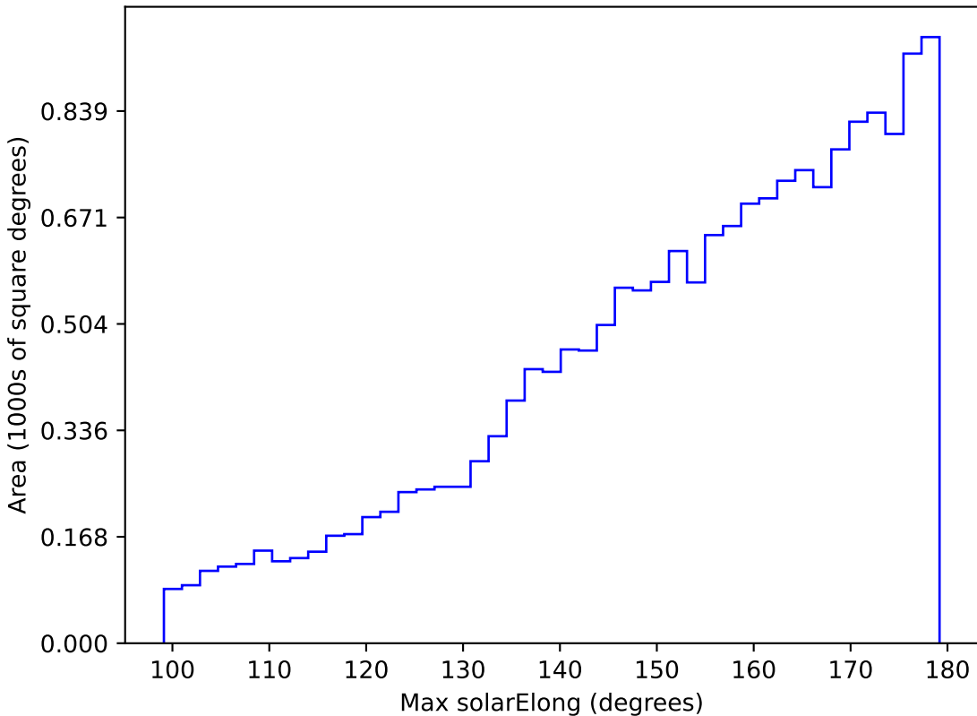
weather_cloudso16v3.4_10yrs WFD g band: Max solarElong
