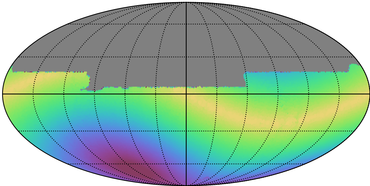
weather_cloudso16v3.4_10yrs All sky y band: Max solarElong
