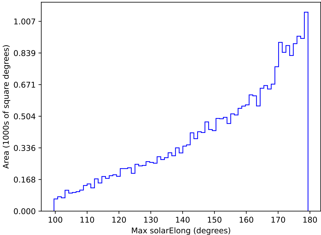
weather_cloudso16v3.4_10yrs All sky i band: Max solarElong
