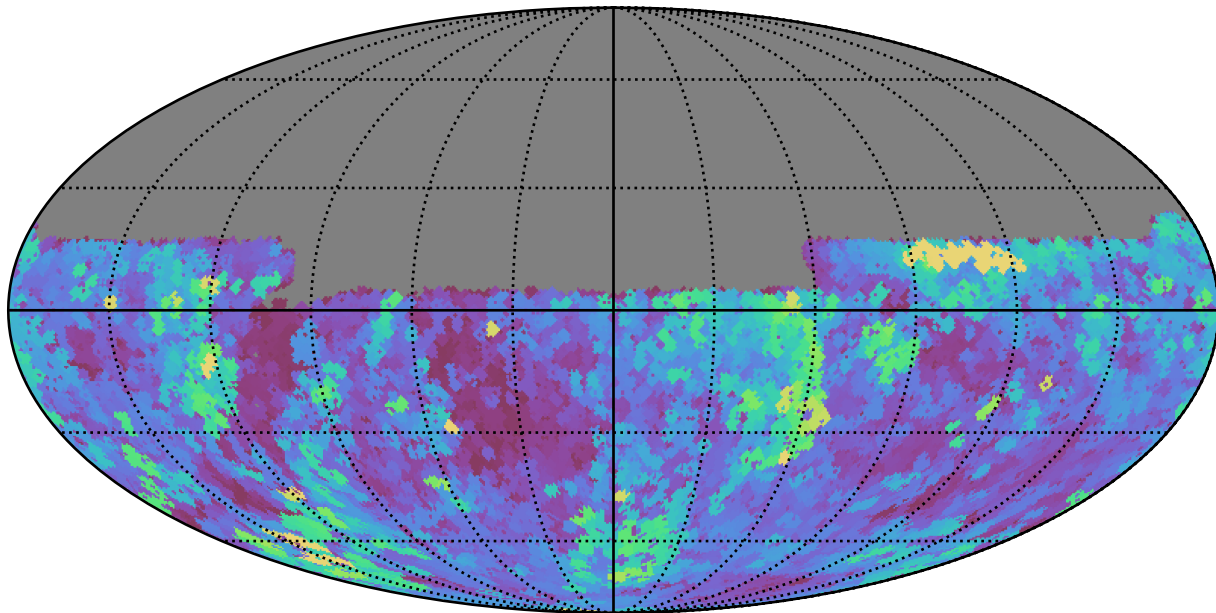
weather_cloudso16v3.4_10yrs Yr 1 y band: Max seeingGeom
