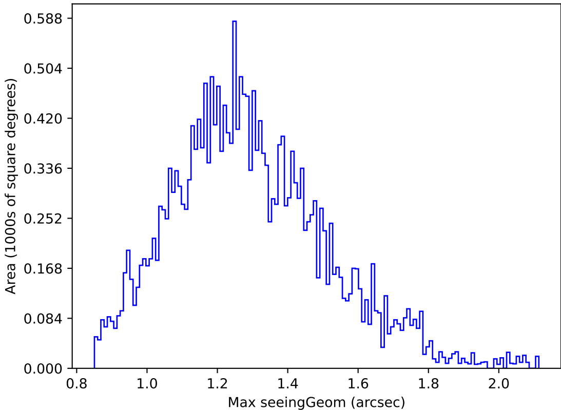
weather_cloudso16v3.4_10yrs Yr 1 y band: Max seeingGeom
