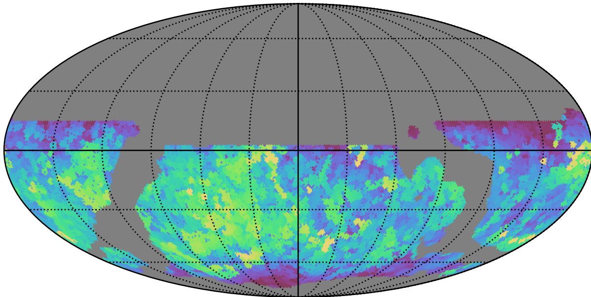
weather_cloudso16v3.4_10yrs WFD z band: Max saturation_mag
